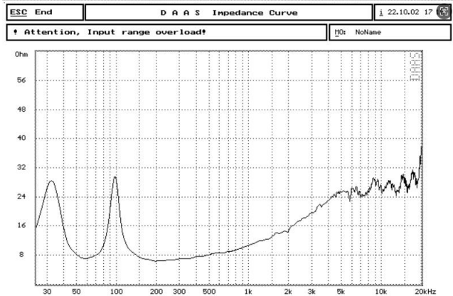
Impedance (Subwoofer)
